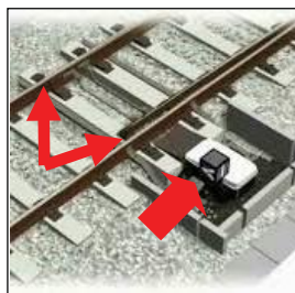
(figura 4) Indicatore e punta deviatore
